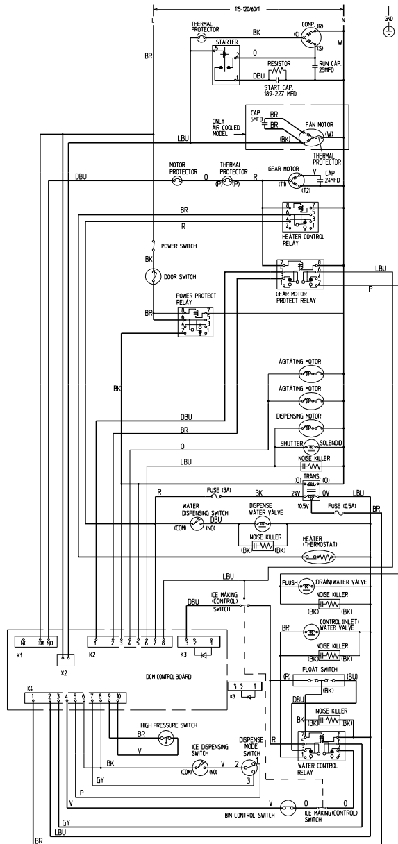
DCM-750BAH, DCM-750BWH
